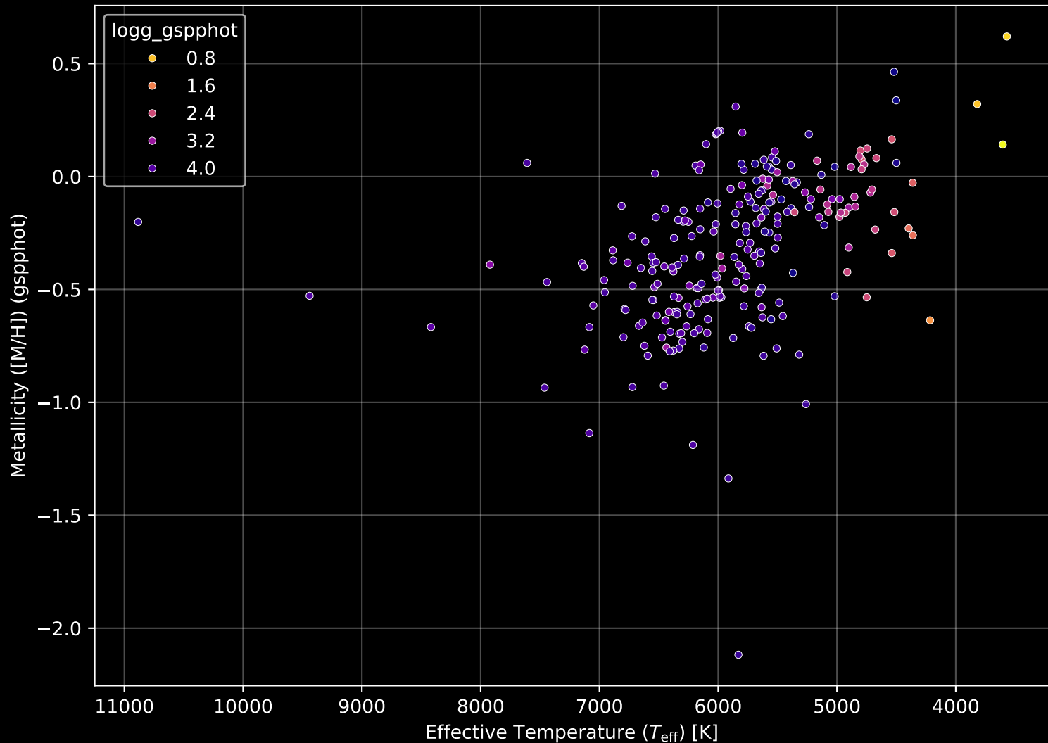
GALAH DR4 Field: [7166] Stellar Population Parameters (n= 248)
