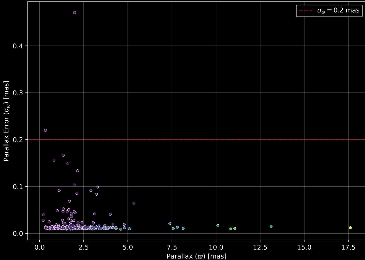
GALAH DR4 Field: [7166] Parallax Quality (n= 248)
